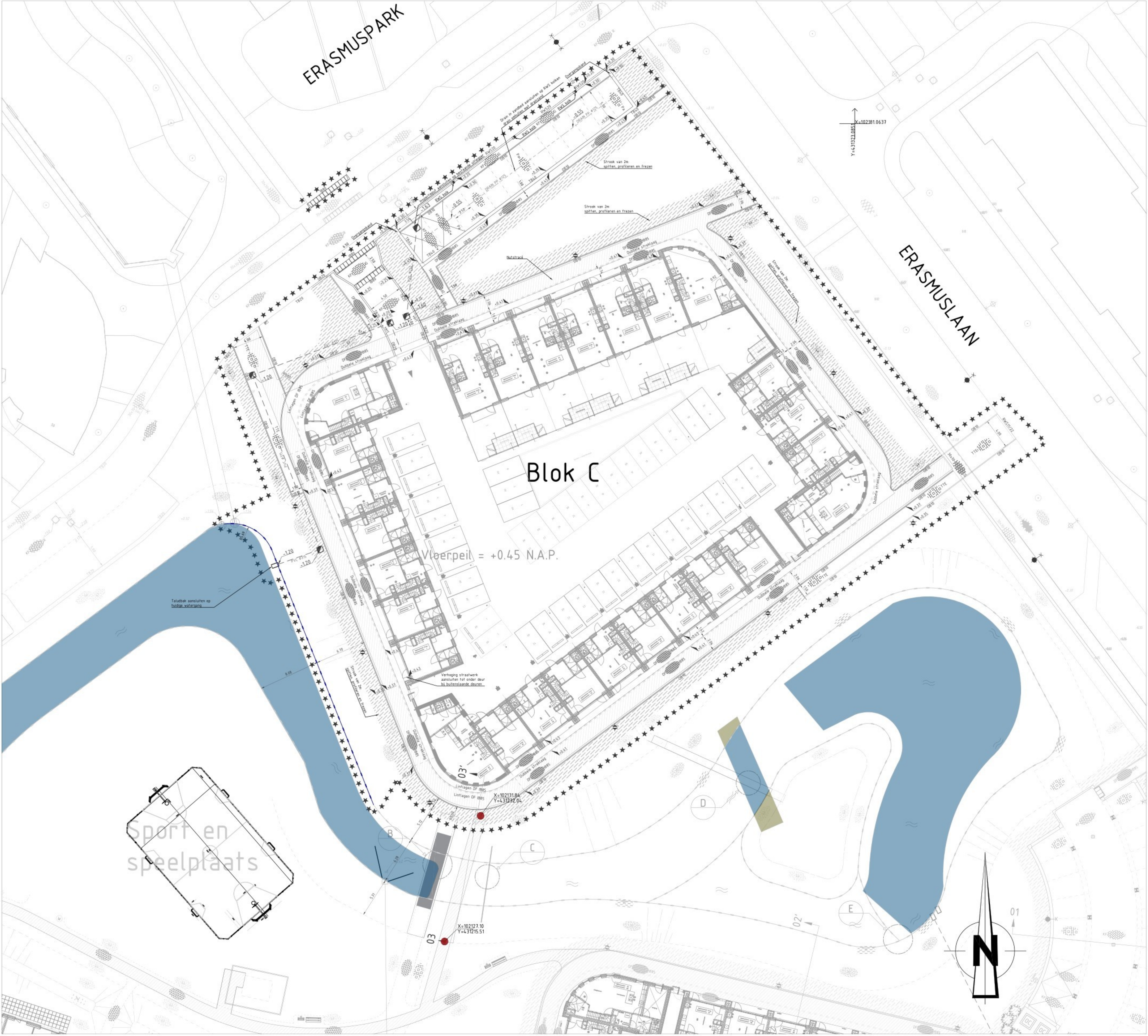
NIEUWE SITUATIE SCHAAL 1:200
