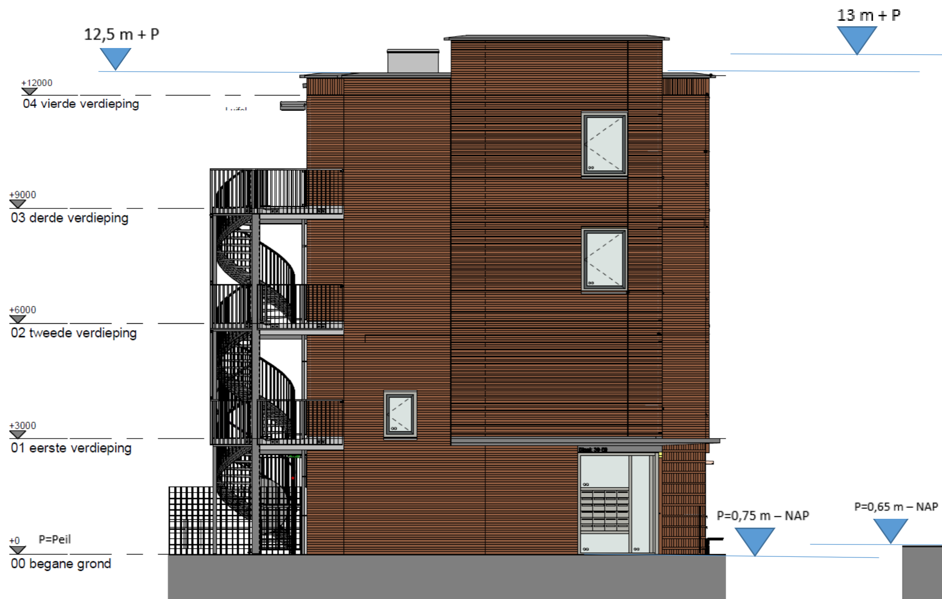
Kopgevelaanzicht nieuwbouw appartementengebouw
