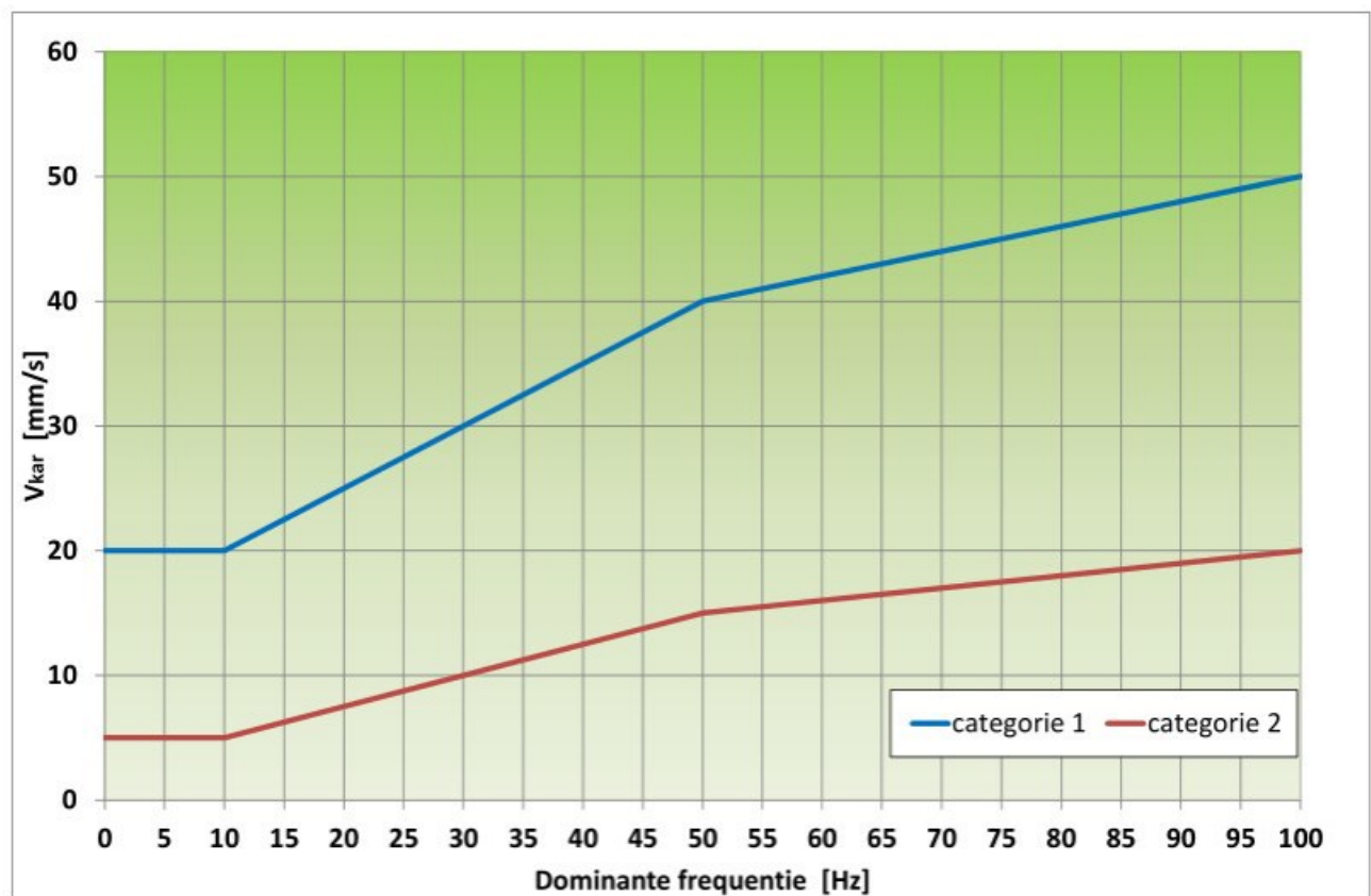
Figuur 10.3 Karakteristieke grenswaarden begane grond voor de twee categorieën bouwwerk.
