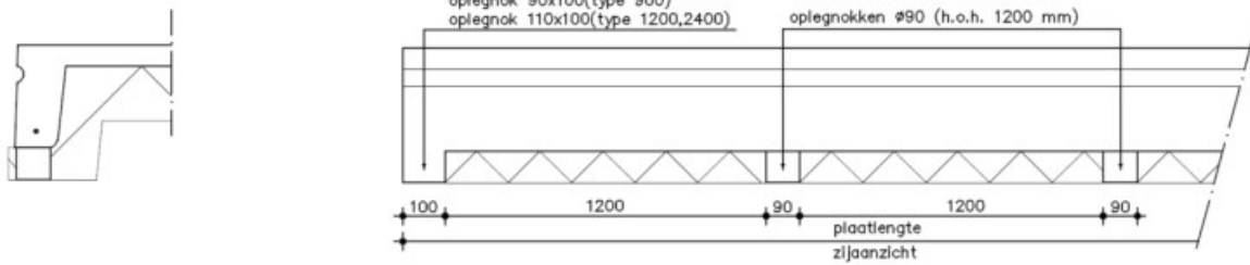
oplegnokken t.p.v. voorspanrib type 900,1200 en 2400
