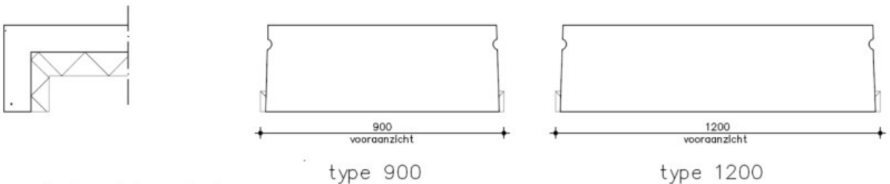
ongeisoleerd kopschot
