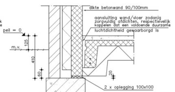
betondetail 5
