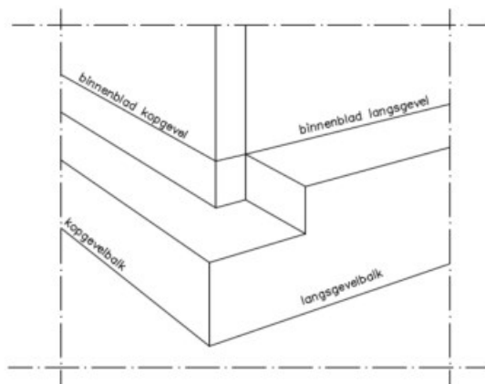
kopgevelspouw dieper dan langsgevelspouw
