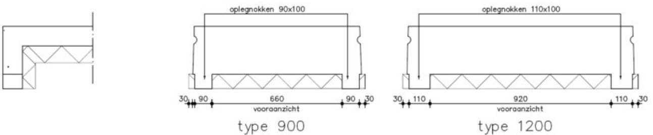
geisoleerd kopschot met oplegnokken
