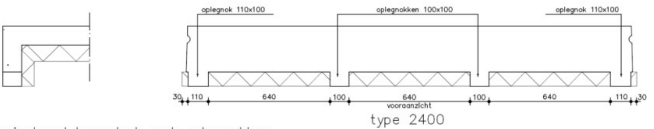
geisoleerd kopschot met oplegnokken
