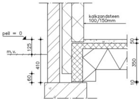
kalkzandsteendetail 1A
