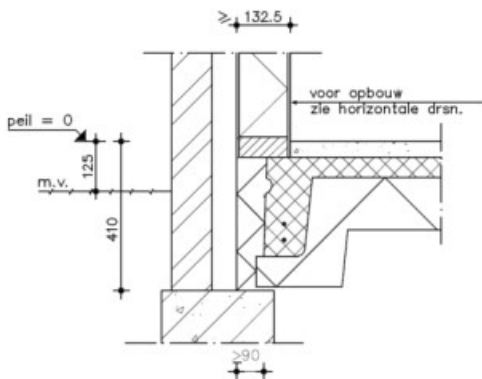
detail 6 –houten binnenspuwblad
