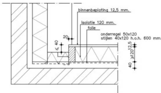
horizontale aansluiting houten binnenspuwblad
