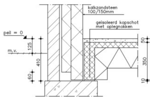
kalkzandsteendetail 1B
