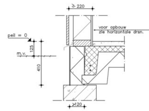
detail 6 –vliesgevel
