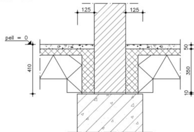
indien wand woningscheidend zie tabel 5 detail 4Ba
