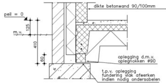
betondetail 6
