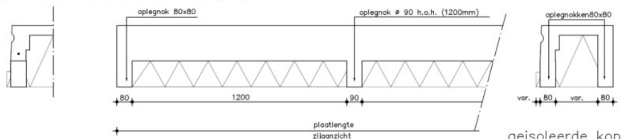
oplegnokken voorspanrib type 400
