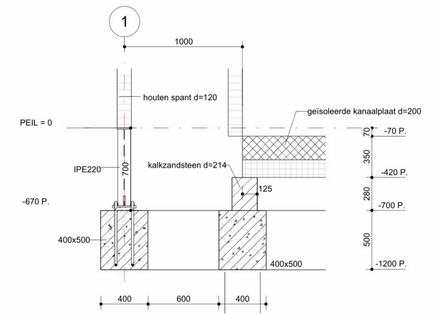
Detail 08 schaal 1:20
